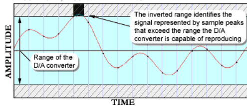
D/A converter range
